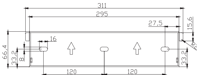
Dimensiones del soporte del modelo GH-I 2M Style y GH-I 2M-15 Style (3 kW - 6 kW)
