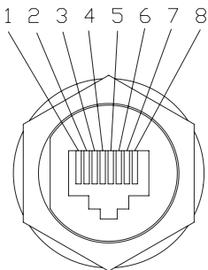
Clavija RS485
