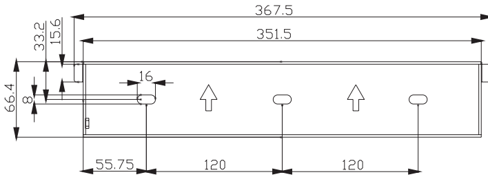
Dimensiones del soporte del modelo GH-I 2M Style y GH-I 2M-15 Style (7 kW - 8 kW)
