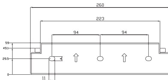
Dimensiones del soporte del modelo GH-I 1M Style y GH-I 1M-15 Style
