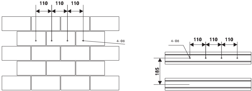
Dimensiones de los agujeros de perforación del inversor GH-IT 2M ADVANCED
