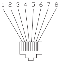
CLAVIJA RS485
