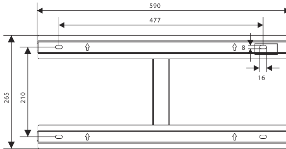
Dimensiones del panel trasero del inversor GH-IT 3M y 4M ADVANCED
