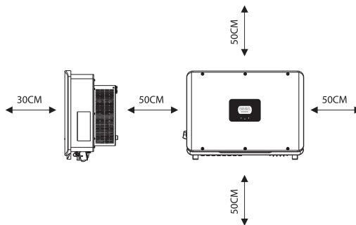
Espacio mínimo
