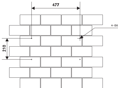
Dimensiones de los agujeros de perforación del inversor GH-IT 3M y 4M ADVANCED
