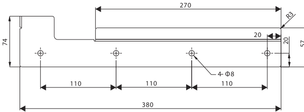
Dimensiones del panel trasero del inversor GH-ITH 2M ADVANCED
