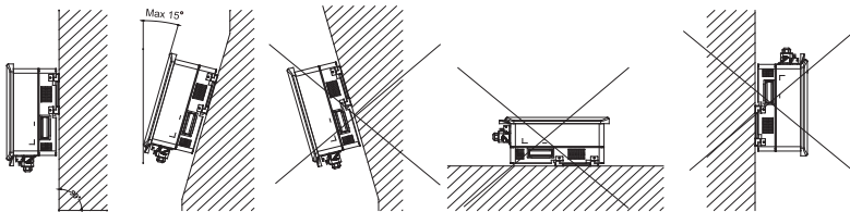
Posición de montaje del inversor
