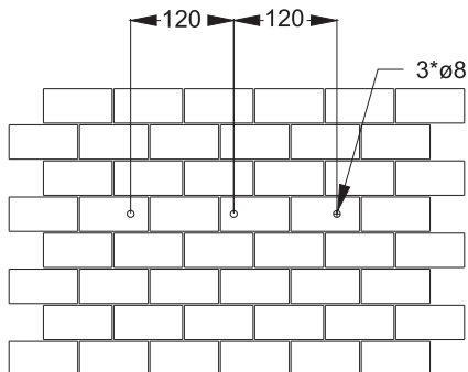
Dimensiones de los agujeros de perforación del inversor GH-IT 2M ADVANCE
