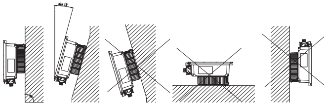
Posición de montaje del inversor
