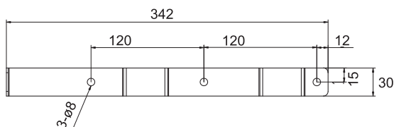
Dimensiones del panel trasero del inversor GH-IT 2M ADVANCE
